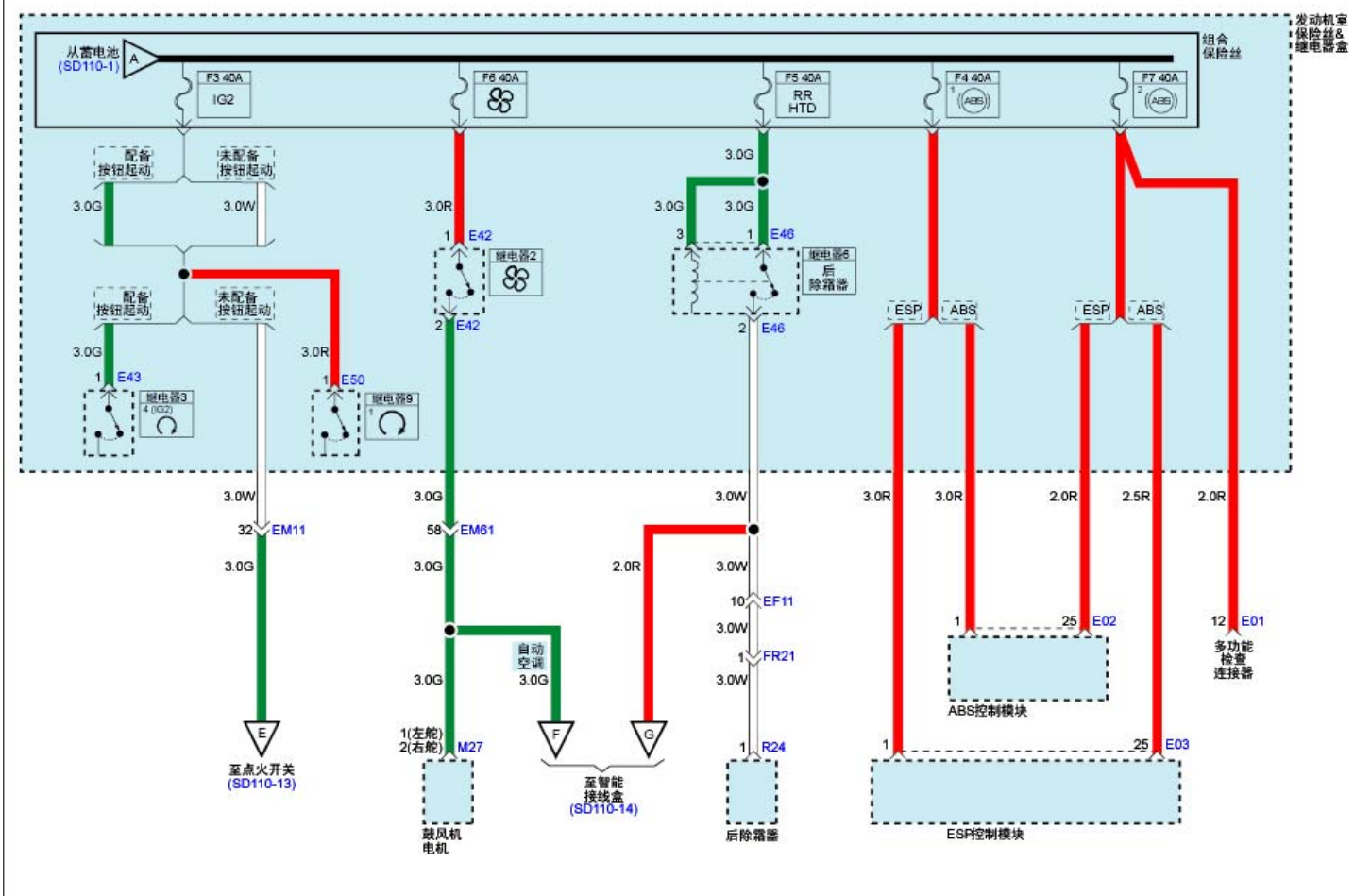
电源分布(2)
